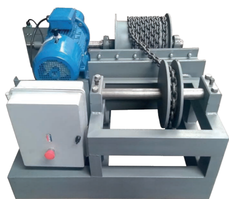
GUINCHE DE IZAJE BOVINO
