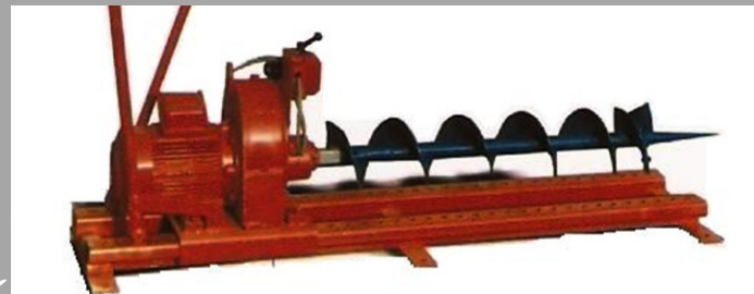
TME 5,5 TUNELERA CON MOTOR A ELÉCTRICO TRIFASICO DE 5,5HP CON CAPACIDAD DE HASTA 0,30m DE DIAM. POR HASTA 20ML DE LARGO
