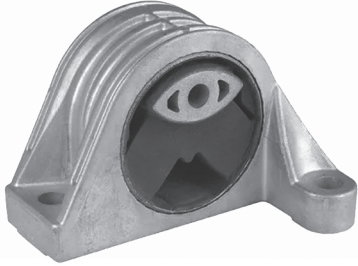
Código: 50200 Modelo: DUCATO 2.8 2.3 N° Original: 1335129080 Soporte de motor derecho
