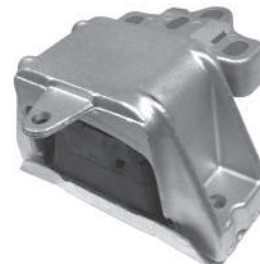
Código: 90048 Modelo: GOLF 1.6 - A4 - A8 Nº Original: 1J0.199.555.BD Soporte motor lado izquierdo
