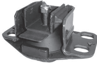
Código: 80146 NO HIDRAULICO Modelo: KANGOO Nº Original: 7700434320 Soporte de motor derecho (no hidráulico)
