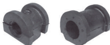
Código: 10006 Modelo: CIVIC 2001 Een adelante Nº Original: 51306-SSJ-003 Buje barra estabilizadora delantero central o 24 mm
