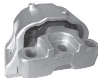
Código: 90045 NO HIDRAULICO Modelo: GOLF 1.6 - BORA - NEW BEETLE Nº Original: 1J0.199.262.BE Soporte motor no hidráulico lado derecho
