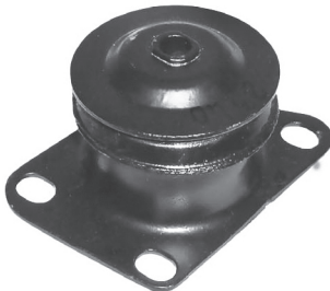
Código: 50161 Modelo: PALIO - SIENA AÑO 2001 en Adelante Nº Original: 51709049 Soporte de motor lado caja
