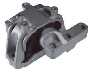
Código: 90082 HIDRAULICO Modelo: VENTO - PASSAT Nº Original: 1K0.199.262 Soporte de motor derecho
