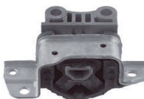
Código: 50199 Modelo: QUBO-FIORINO QUBO Nº Original: 51821084 Soporte de motor derecho
