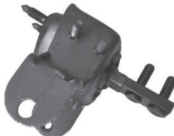
Código: 70168 HIDRAULICO Modelo: ESCORT Nafta Nº Original: 95AB-6038-EF Soporte motor lateral hidráulico
