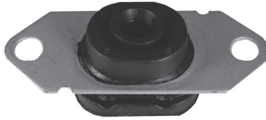
Código: 80213 Modelo: MEGANE 2 K4M Nº Original: 8200352861 Soporte de motor izquierdo
