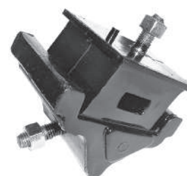
Código: 70134 Modelo: F100 Diesel MAXION Nº Original: 96TU6038AA Soporte de motor delantero
